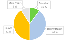
Haematococcus pluvialis
