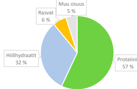
Dunaliella salina
