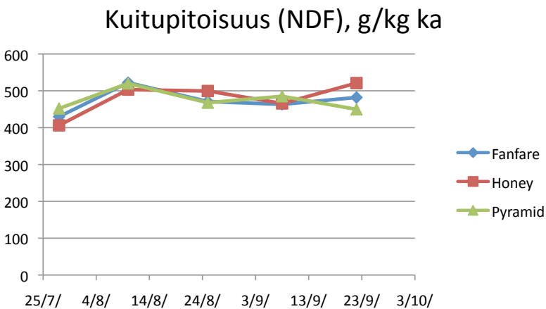
Kuva 21. Kuitupitoisuus.
