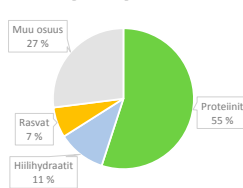
Spirulina platensis
